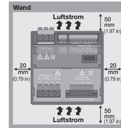
Abb. Einbaulage Rückansicht UMG 96-PQ-L
